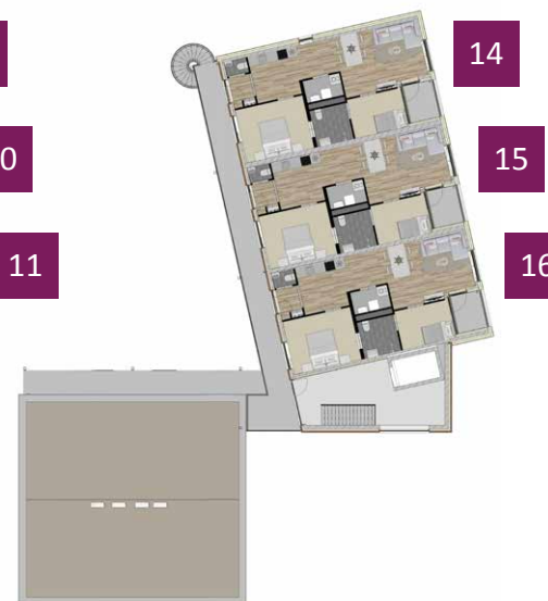
3 de verdieping
